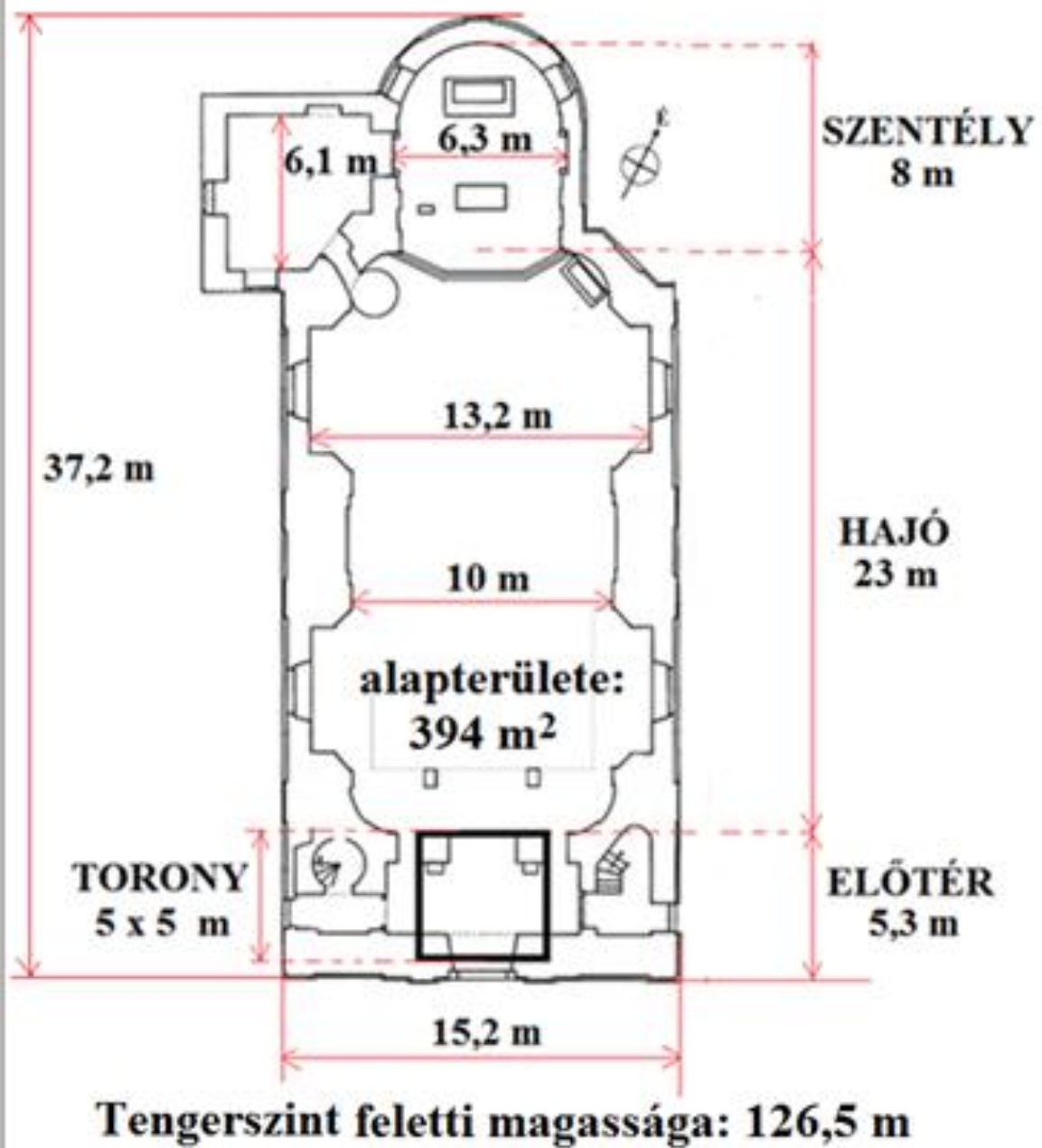
A NYÚLI TEMPLOM MÉRETEI
